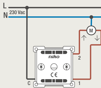
170-55901 / 170-35901 DRAAISCHAKELAAR 1 - 0 - 2 VOOR ROLLUIKEN IMPULSGEVER MET DRAAIBEDIENING (niet voor parallelwerking)
